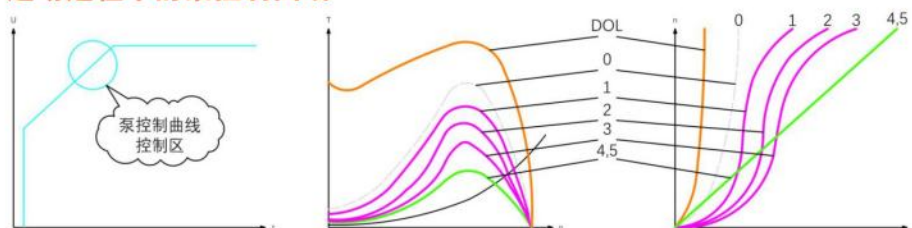
图九、起动过程中的泵控制曲线
