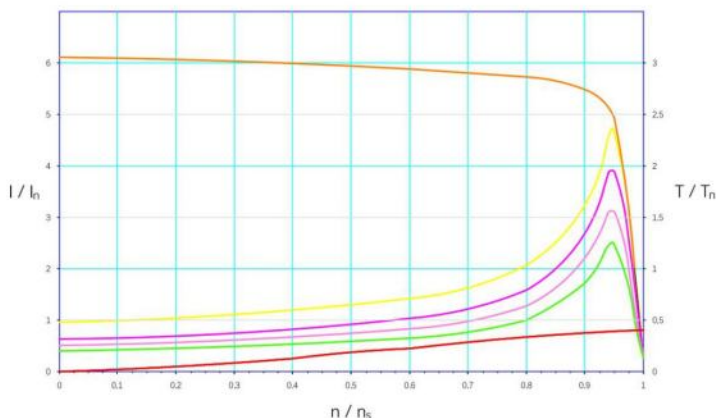
图九、使用MDMVS控制电动机起动
