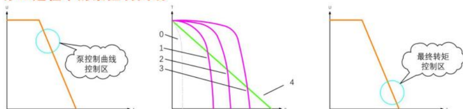
图十、停止过程中的泵控制曲线
