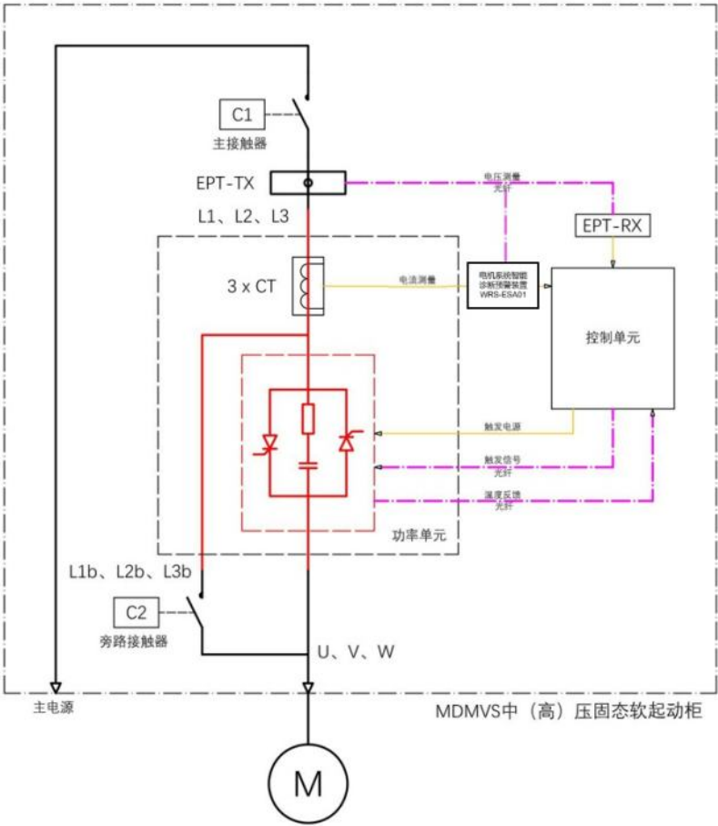
图十二、MDMVS 中(高)压 固态软起动柜系统框图
