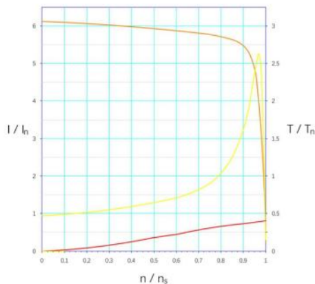
图八、电动机全压起动
