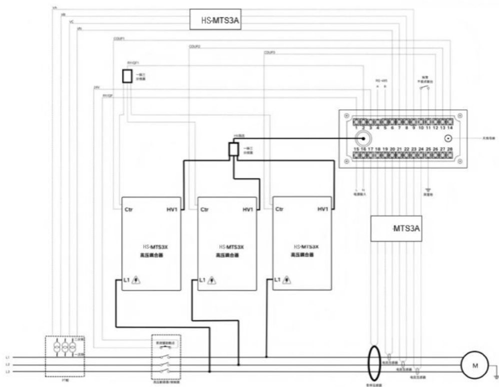
设备接线图（三相绝缘）
