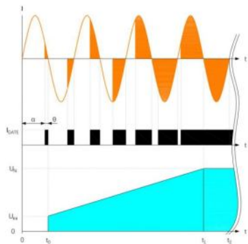
图七、MDMVS移相触发原理
