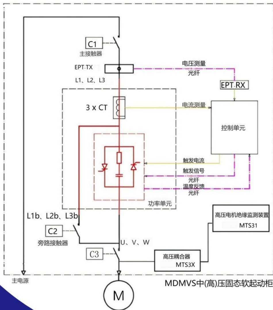
图十、MDMVS中(高)压固态软起动柜系统框图
