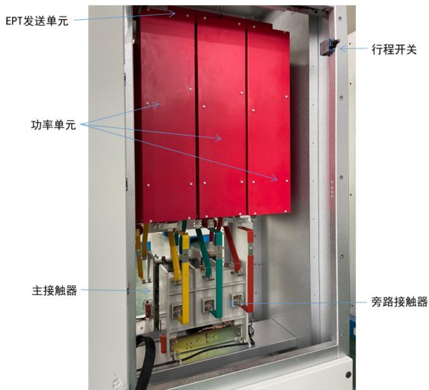
图四、MDMVS中高压固态软起动柜高压舱室
