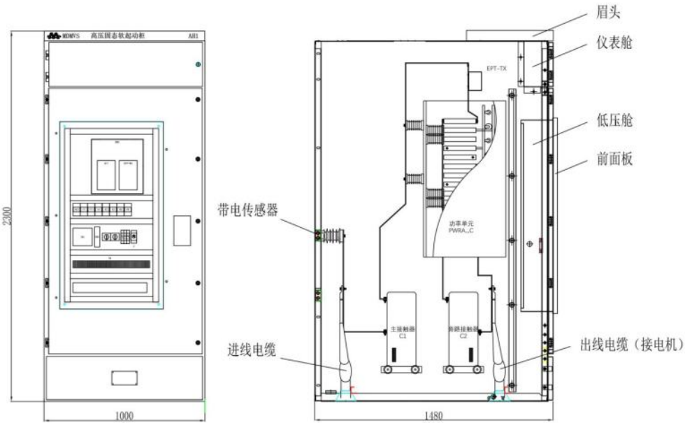
图六、MDMVS结构图
