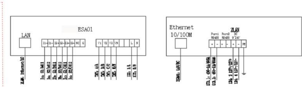
设备接线图
