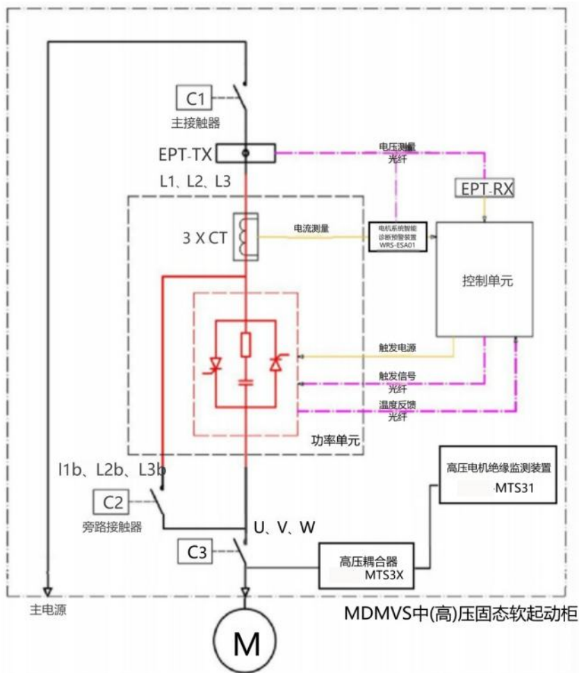
图十一、MDMVS中(高)压固态软起动柜系统框图
